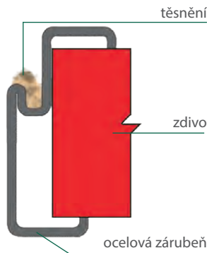
PROFIL OCELOVÉ ZÁRUBNĚ PRO DPB2
