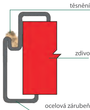
PROFIL OCELOVÉ ZÁRUBNĚ PRO DPB 3
